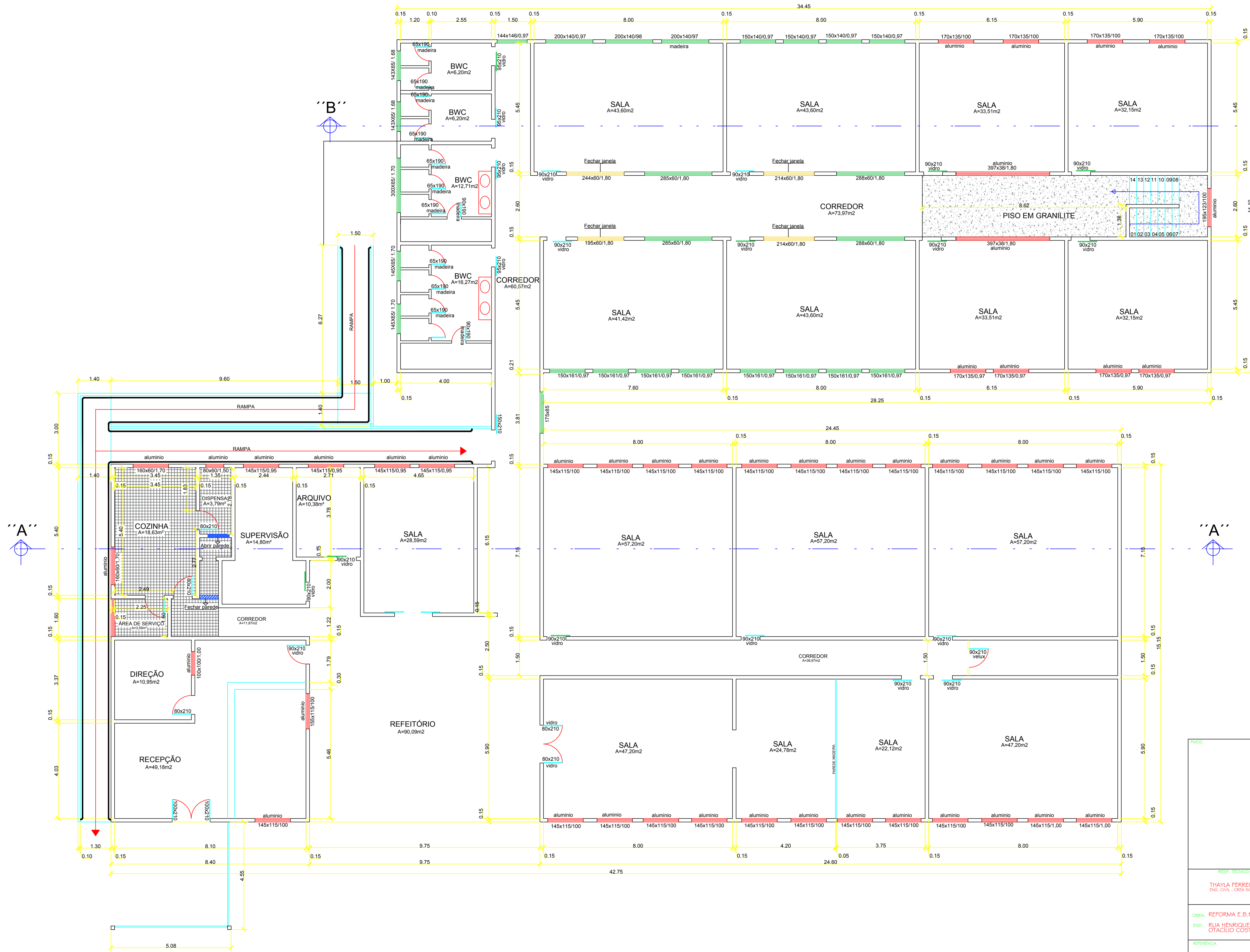
PLANTA BAIXA PAV. TÉRREO ESC:1/50
