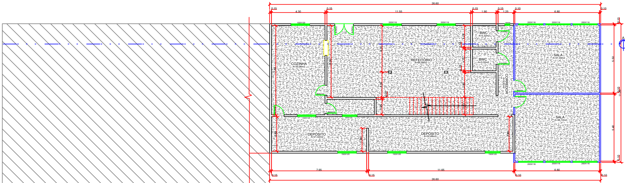
PLANTA BAIXA SUB SOLO esc:1 / 50 área 287,94M2
