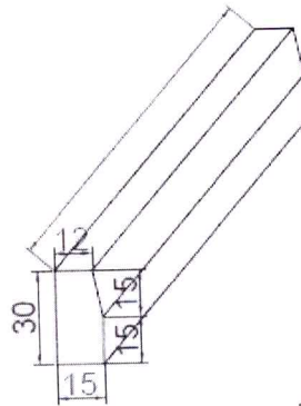
Detalhe do meio fio
