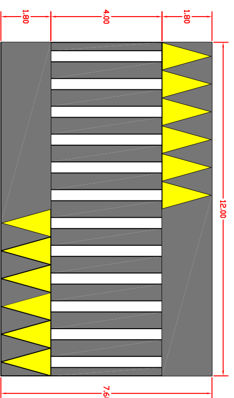
PLANTA BAIXA
