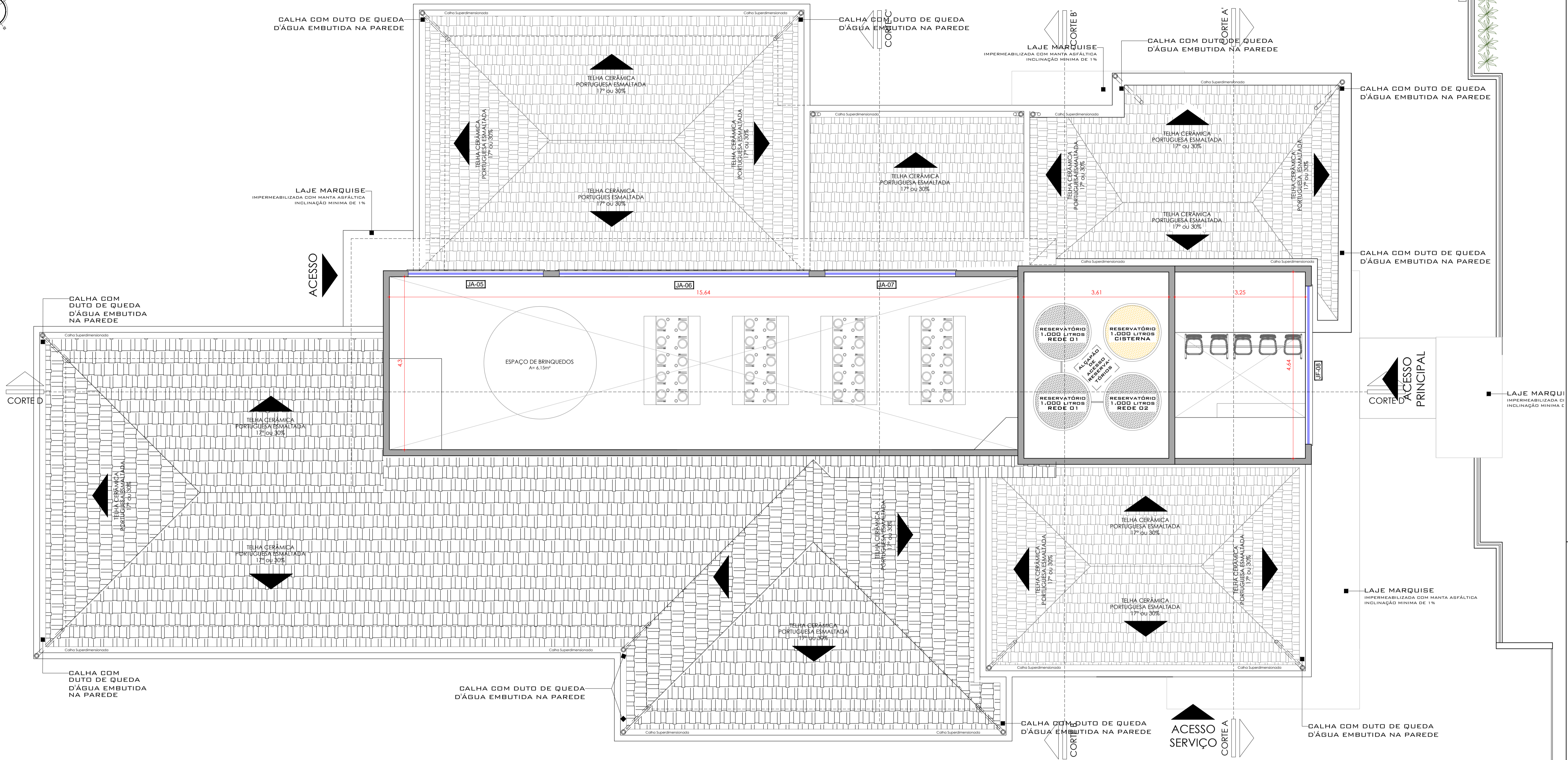
PLANTA BAIXA RESERVATÓRIO E PÉ DIREITO DUPLO
