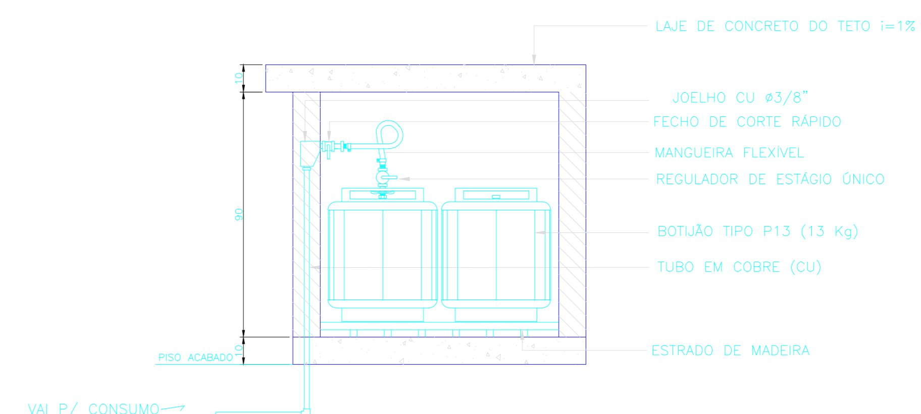
DETALHE ABRIGO P/ GÁS (2 x P 13) SEM ESCALA
