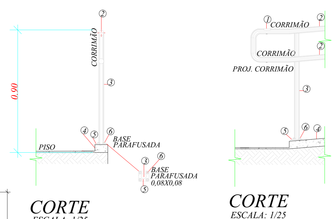
CORTE ESCALA: 1/25
