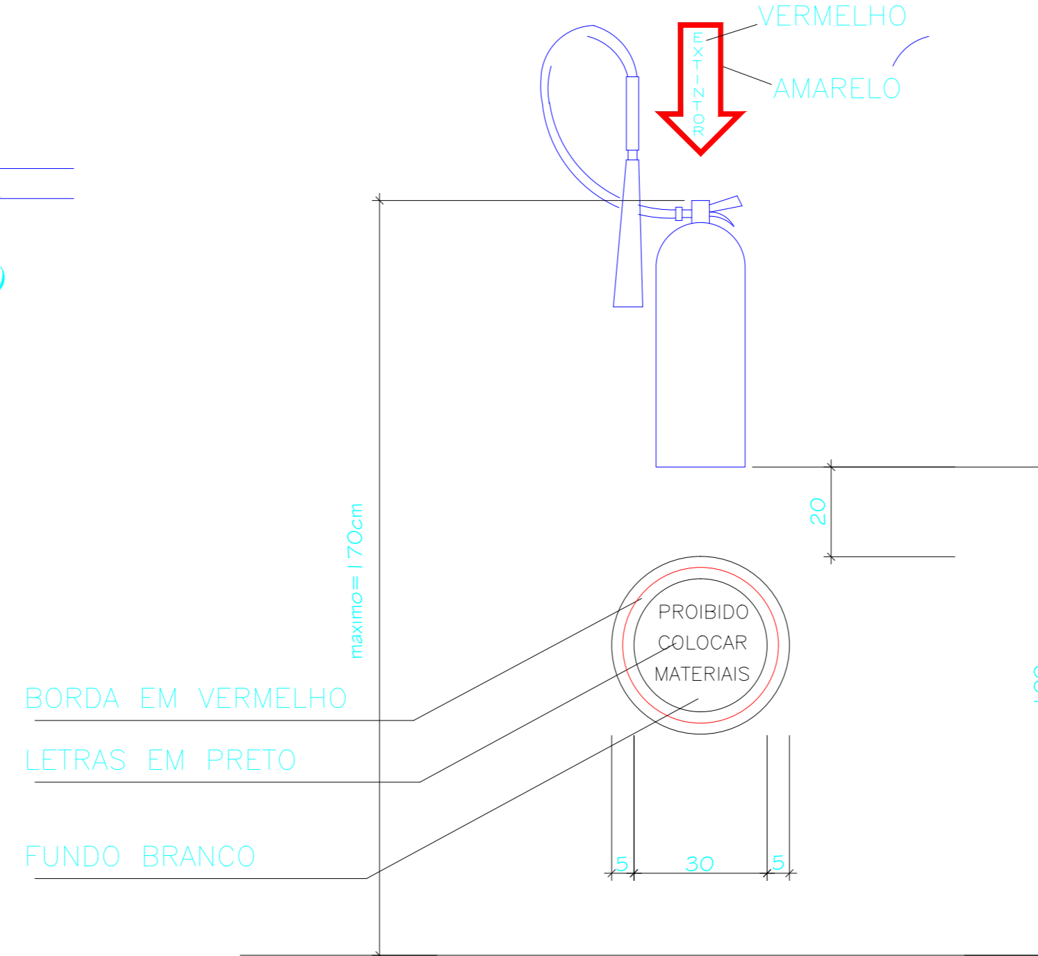
DET. EXTINTOR DE INCENDIO SEM ESCALA
